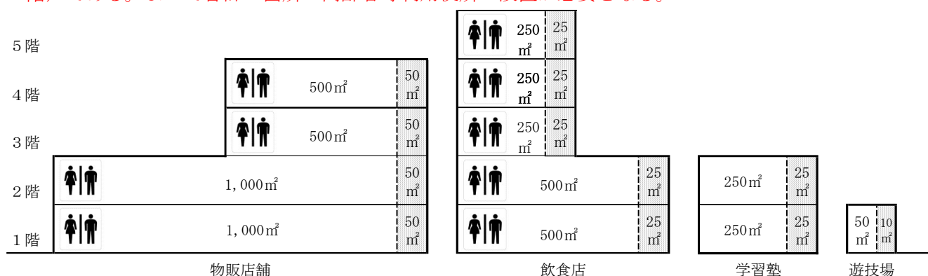
図15 便所を共用しない場合の高齢者等利用便所の配置
