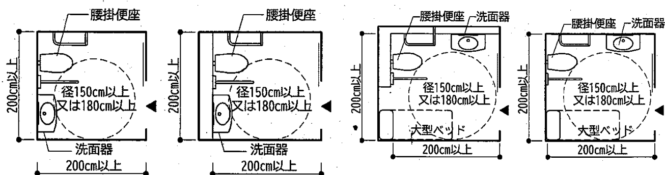
図11 水洗設備の配置と車椅子使用者便房の大きさの例
