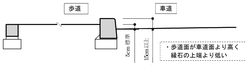
図 30 歩道断面
