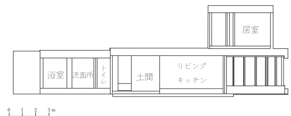
断面図 S=1/100
