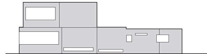
立面図 S=1/100
