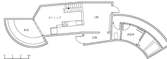
1 階平面図 S=1/100
