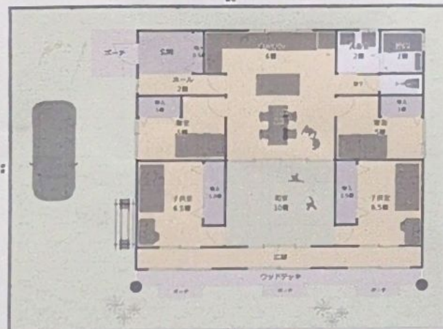
配置図兼1階平面図 S=100
